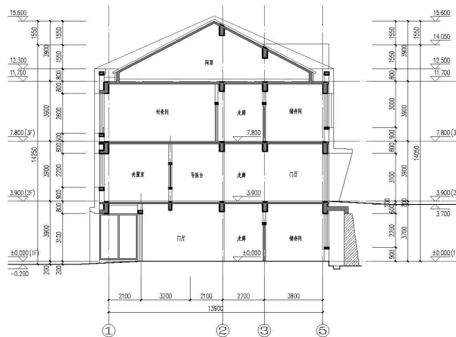
2-2剖面图 1:100
