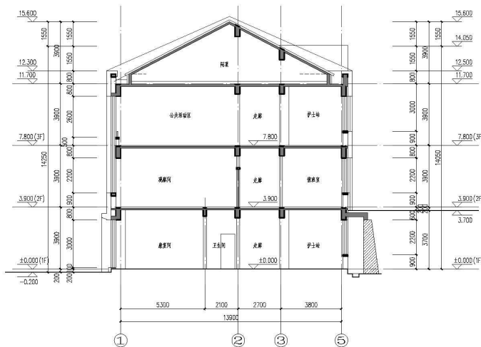
1-1剖面图 1:100
