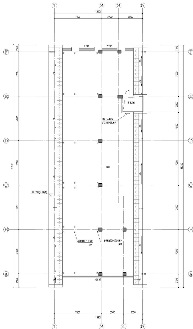
屋顶平面图 1:100
