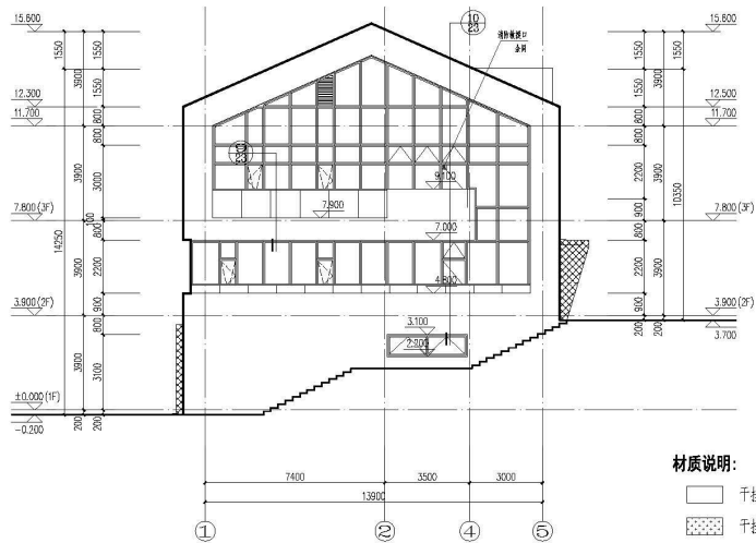
①-⑤ 轴立面图 1:100
