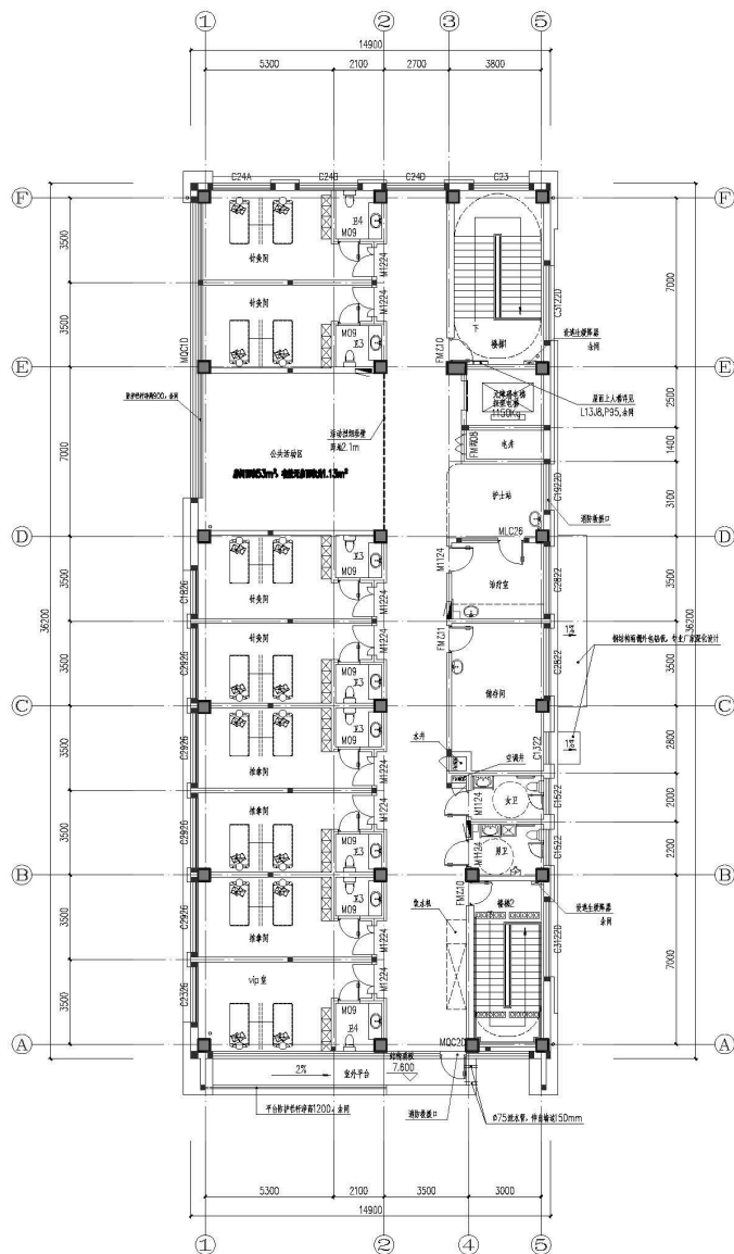
三层平面图 1:100 本层建筑面积556.93平方米 未注明的参照地下室
