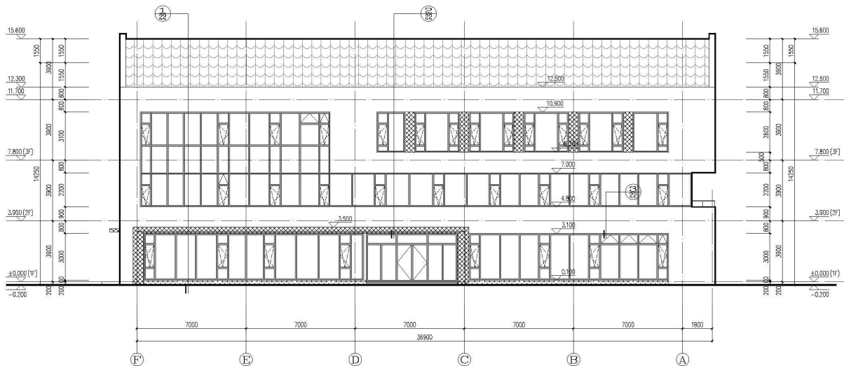
(F')-A 轴立面图 1:100
